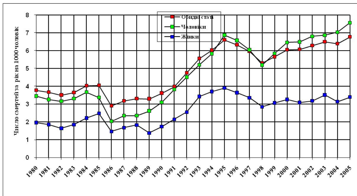
Рис. 3.3. Динаміка змін екзогенної складової коефіцієнтів смертності від усіх причин для чоловічого та жіночого населення, а також для обох статей
