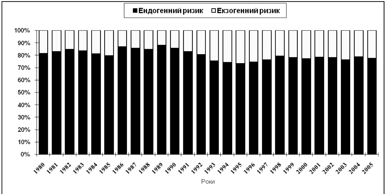
Рис. 3.6. Екзогенні та ендогенні складові (у відсотках) ризику смертності жіночого населення України у 1980 - 2005 рр.
