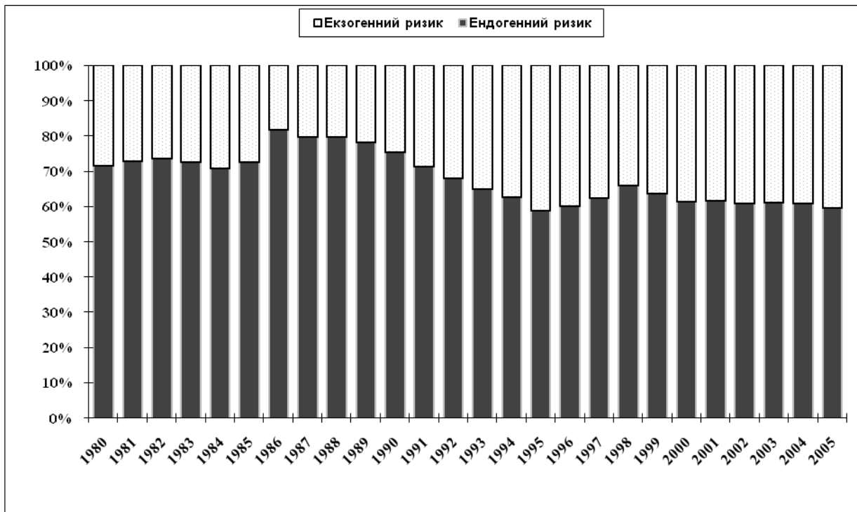
Рис. 3.5. Екзогенні та ендегенні складові (у відсотках) ризику смертності чоловічого населення України у 1980 - 2005 рр.
