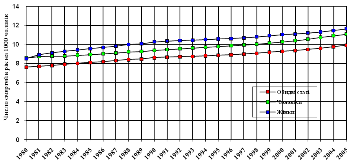
Рис. 3.4. Динаміка змін ендогенної складової коефіцієнтів смертності від усіх причин для чоловічого та жіночого населення, а також для обох статей
