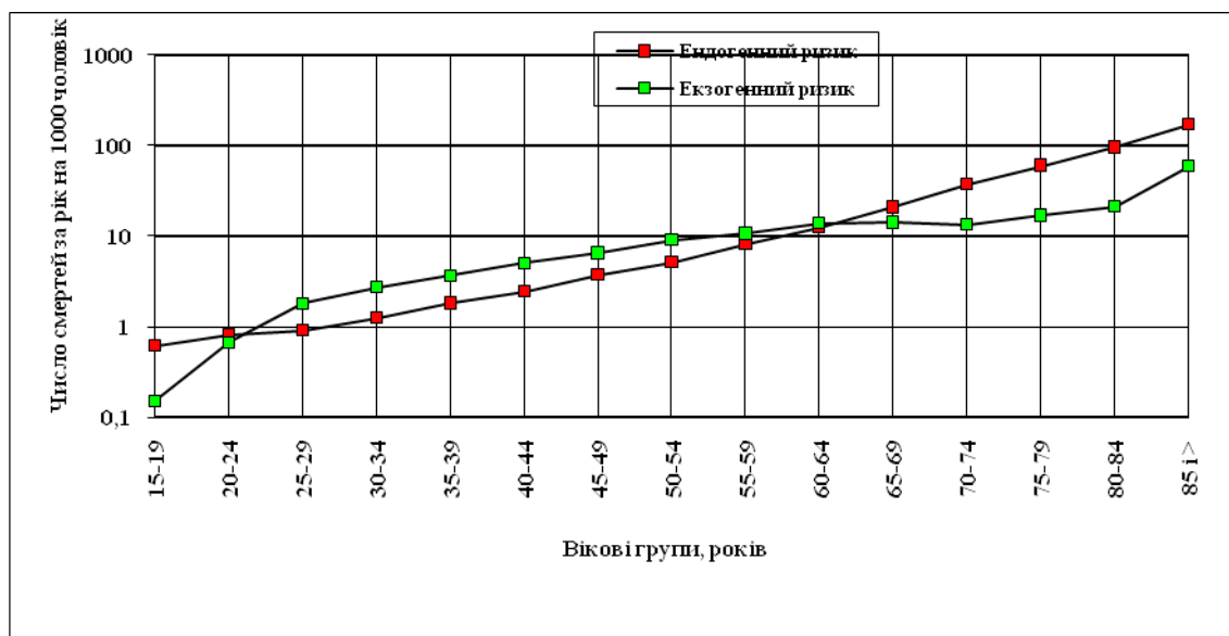
Рис.3.1. Розподіл за віком ендогенної та екзогенної складових ризиків смертності населення України від усіх причин у 2005 році
