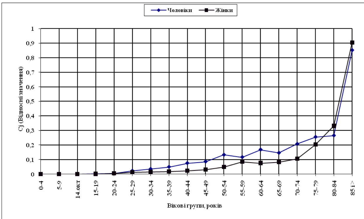
Рис. 3.2. Розподіл за віком екзогенної складової ( C_j ) ризику смертності від усіх причин для чоловічого і жіночого населення України (1980 – 2005 рр.)
