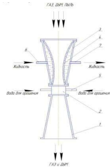
Рис. 4 Пристрій для очищення газів типу труби Вентурі
