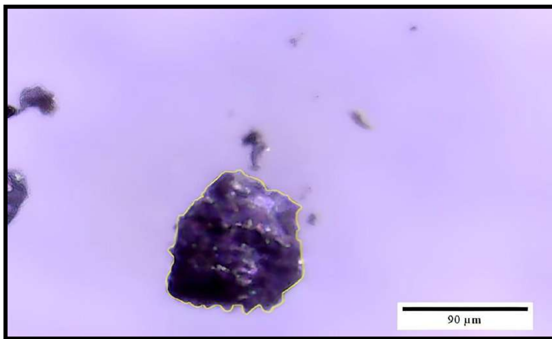
Рис. 1 Зміна поверхні вугільної частинки золи винесення
