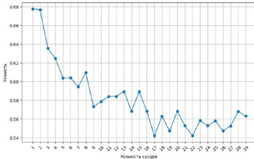
Рис. 2. Залежність точності від кількості сусідів для KNN
