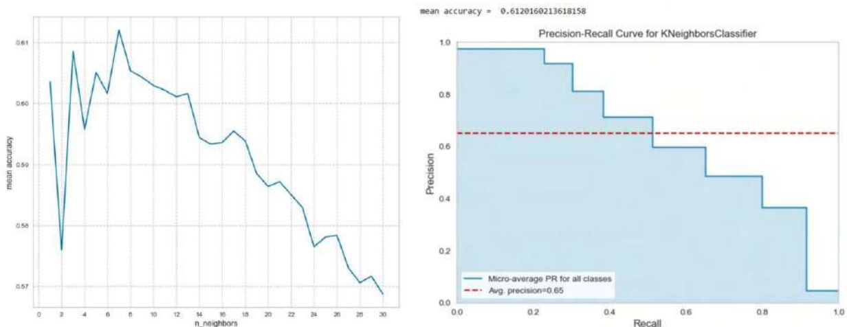
Рис. 11. KNN, перебір кількості сусідів та результати оцінки моделі
