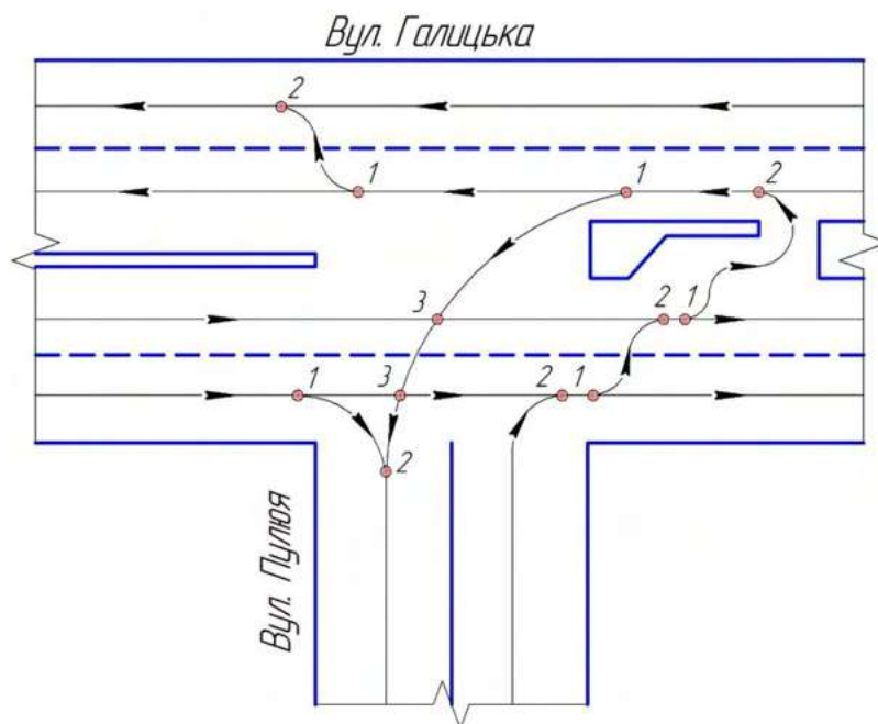
Рис. 2. Запропонована Схема здійснення віднесеного лівого повороту на перехресті вул. Пулюя-Галицька (м. Івано-Франківськ)
