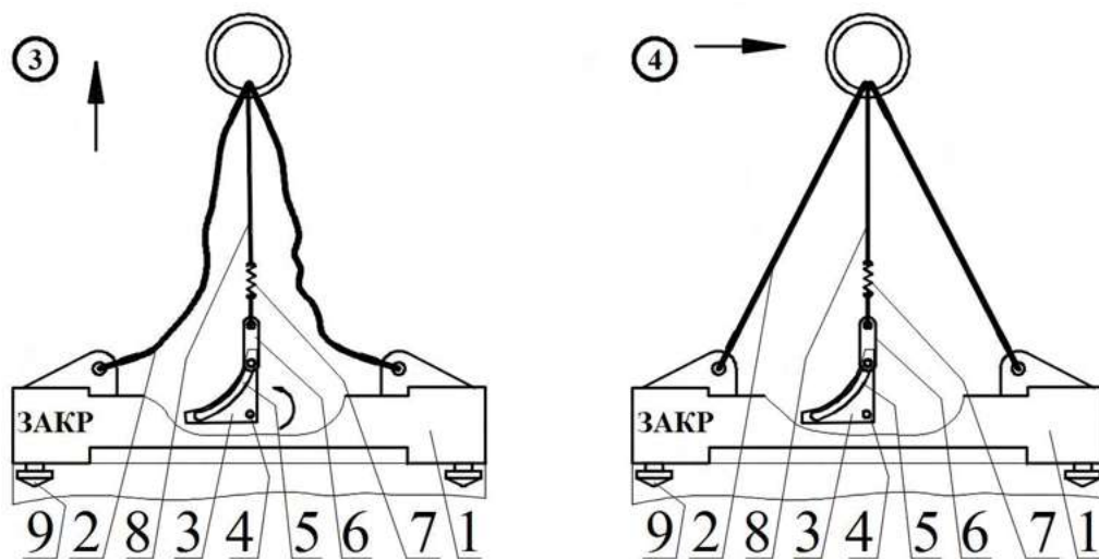
Рис. 3. Схема роботи спеціальних захватів для контейнерів.
