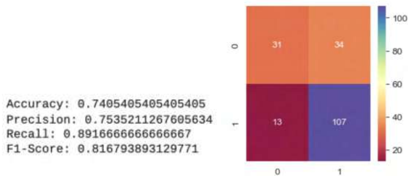
Рис. 7. Результати для дерева рішень
