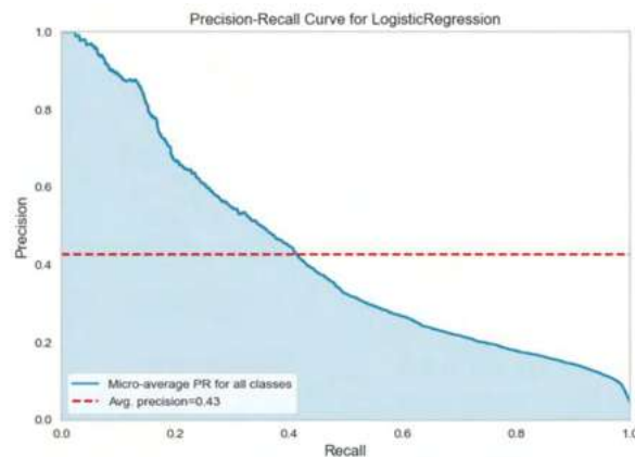
Рис. 10. Логістична регресія, результати
