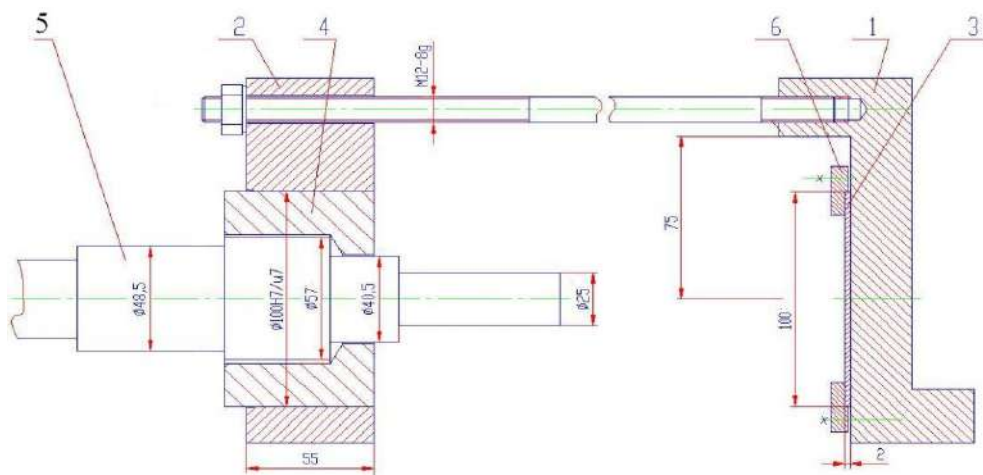
Рисунок 1 – Пристрій для встановлення заготовки
