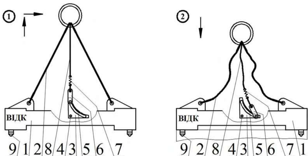
Рис. 2. Схема роботи спеціальних захватів для контейнерів.
