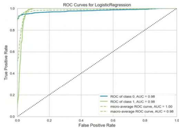
Рис. 14. Логістична регресія, результати
