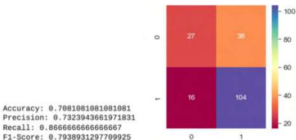
Рис. 6. Результати для логістичної регресії
