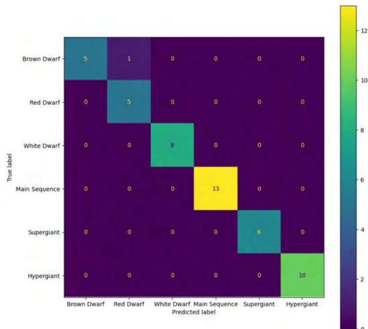
Рис. 5. Матриця невідповідностей для моделі SVM
