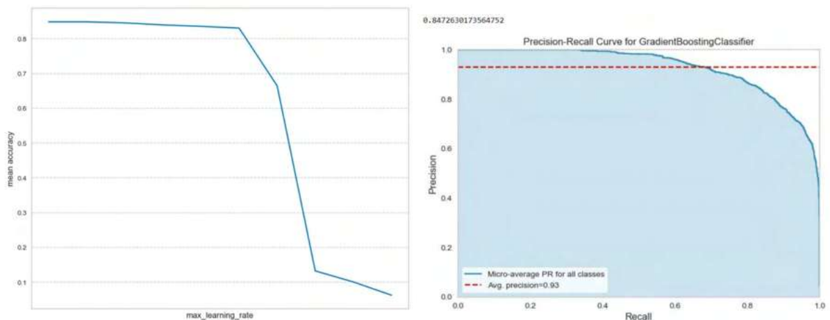
Рис. 13. GBC, підбір параметра та результати
