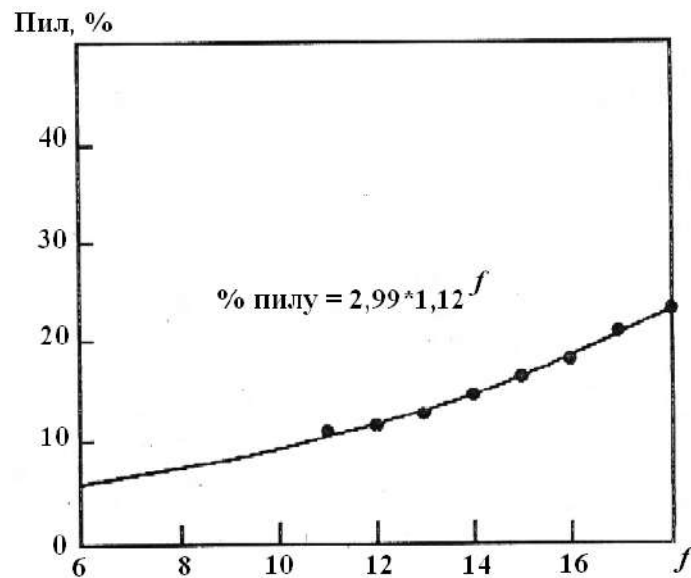
Рис. 1. Залежність кількості кварцового пилу в продуктах вибухового руйнування залізистих кварцитів від міцності порід ( f )
