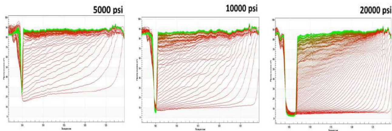
Рис 1. Результати, отримані для емульсії 5000, 10 000, 20 000 psi / 345, 690, 1380 бар після одного проходу через процесор Microfluidizer.
