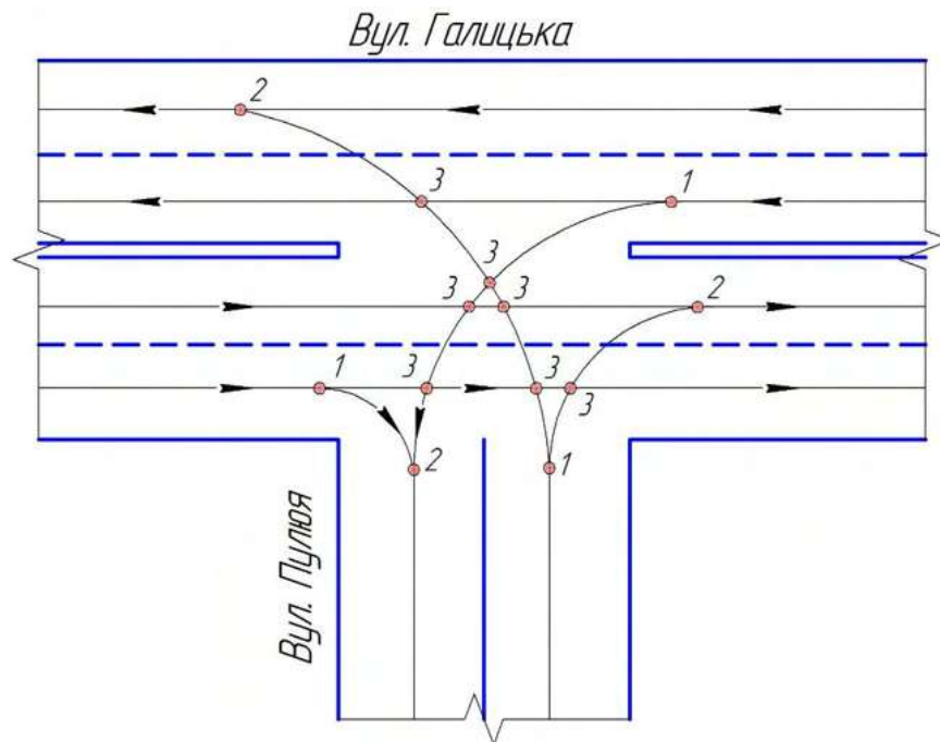
Рис. 1. Існуюча схема здійснення прямого лівого повороту на перехресті вул. Пулюя-Галицька (м. Івано-Франківськ)
