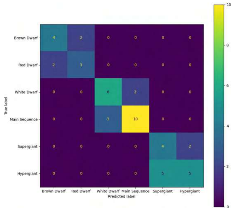
Рис. 3. Матриця невідповідностей для моделі KNN
