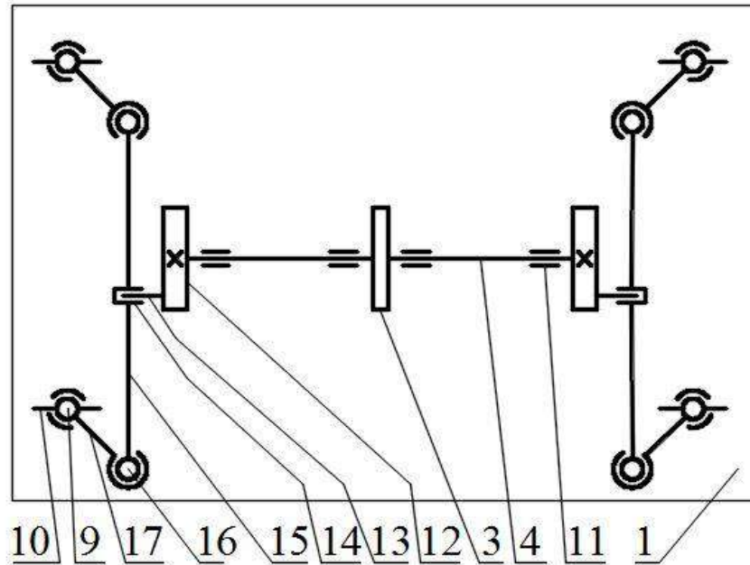
Рис. 5. Кінематична схема пристосування для перевантаження контейнерів (положення відкрито).
