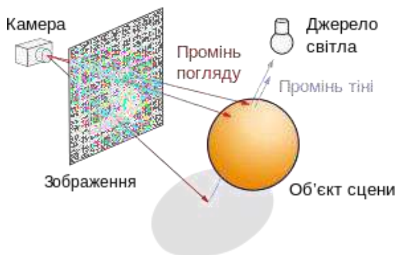
Рис. 1. Принцип роботи алгоритму трасування променів
