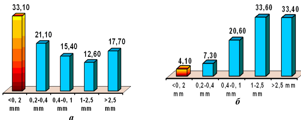
Рис. 2. Гістограми фракційного складу продуктів руйнування гранітів (а) і доломітів (б). Цифри над стовпчиками – вихід фракцій у відсотках
