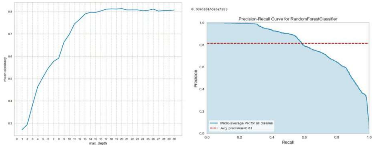
Рис. 12. RFC, перебір висот дерева та результати оцінки моделі
