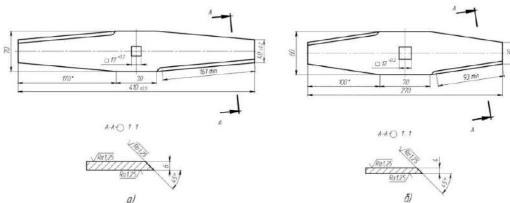
Рис. 1. Розміри ножів: а) основного ножа, б) додаткового ножа
