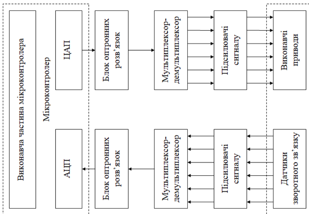
Рис. 1. Структурна схема пристрою керування
