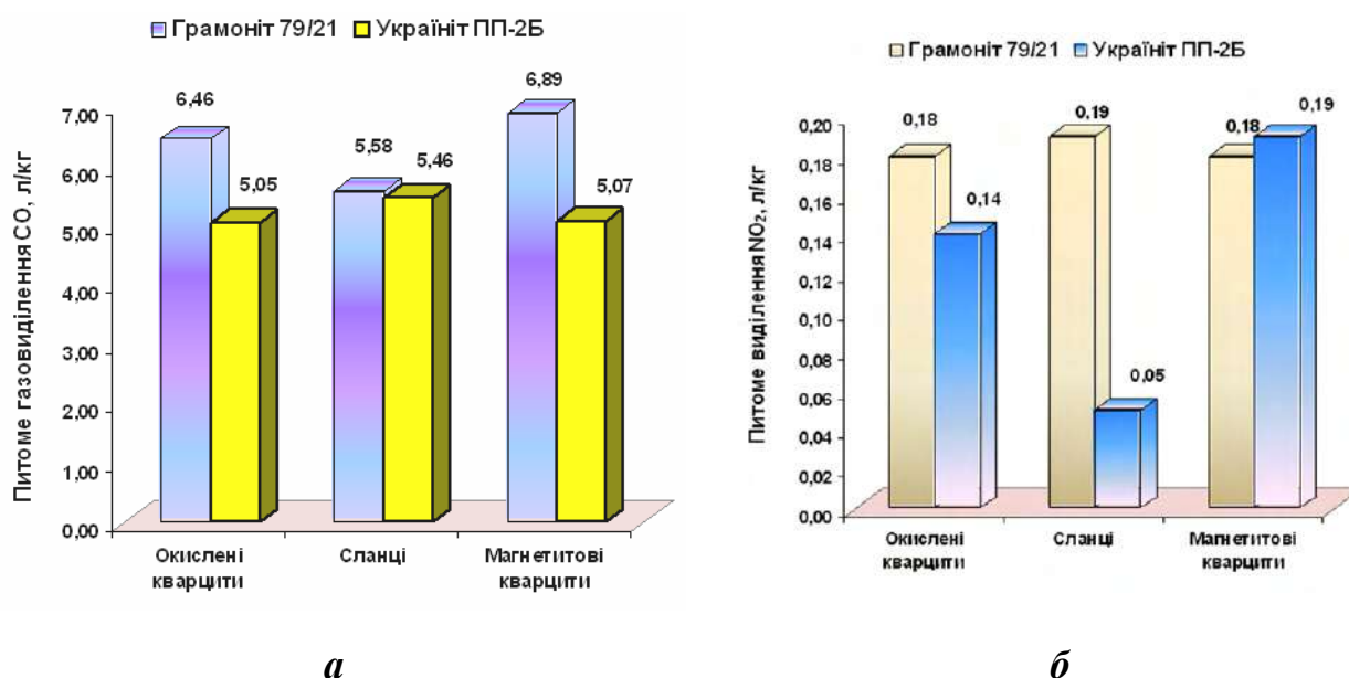
Рис. 3. Гістограми питомого виділення шкідливих газів вибуху в залежності від типів порід, що руйнуються
