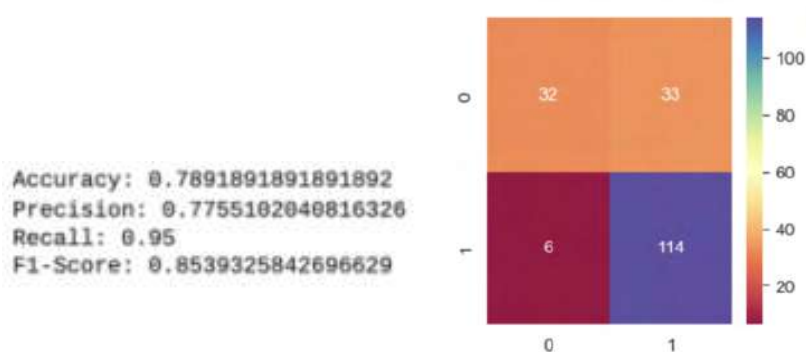
Рис. 8. Результати для випадкового лісу
