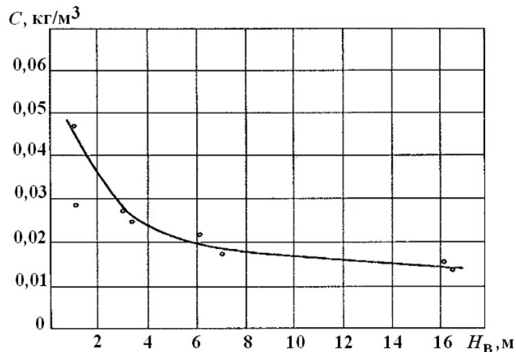
Рис. 4. Залежність питомого пиловидалення під час вибухів від обводненості свердловин
