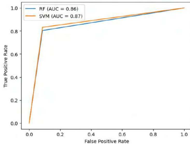
Рис. 6. Порівняння ROC кривих для моделей RF та SVM
