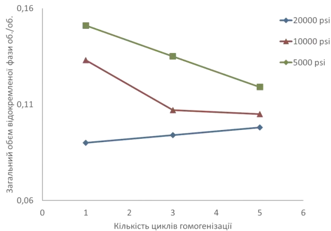
Рис 2. Визначення впливу кількості циклів на співвідношенням загального об'єму рідкої фази, відокремленої після заданого часу центрифугування, до об'єму всієї проби.
