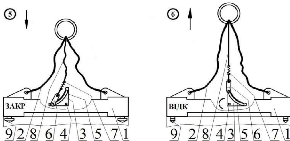
Рис. 4. Схема роботи спеціальних захватів для контейнерів.
